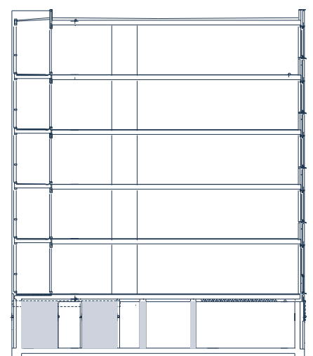
Doorsnede
